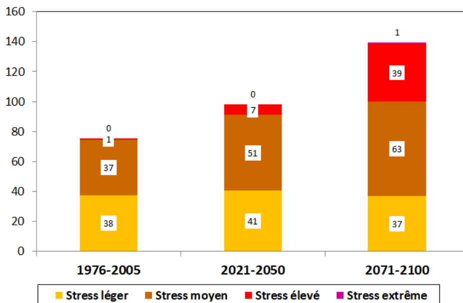
Evolution des classes de THI en nbr de jours par an (médiane par période de 30 ans)
